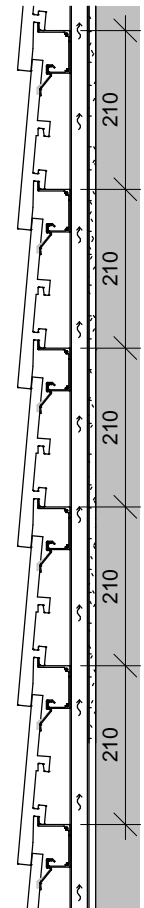
Senkrechter Schnitt 1 : 10
