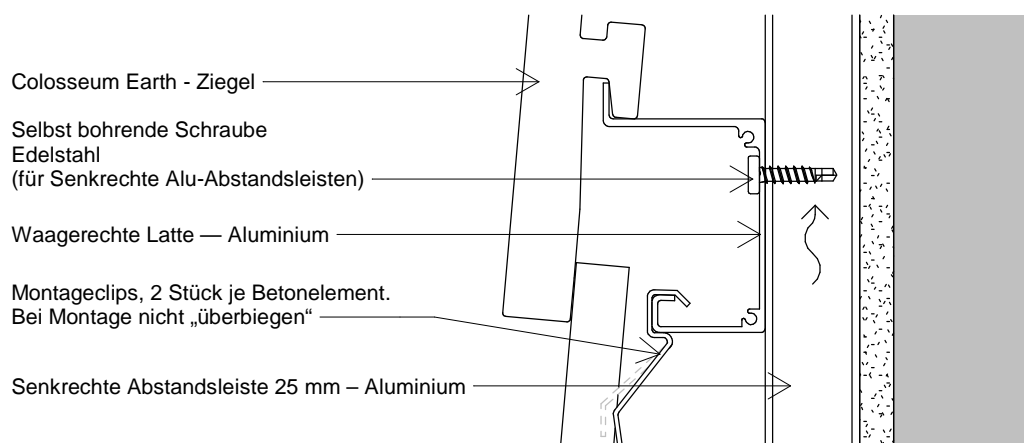
Senkrechter Schnitt 1 : 2
